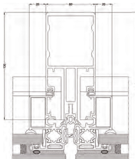
Facciate strutturali Structural curtain walls
