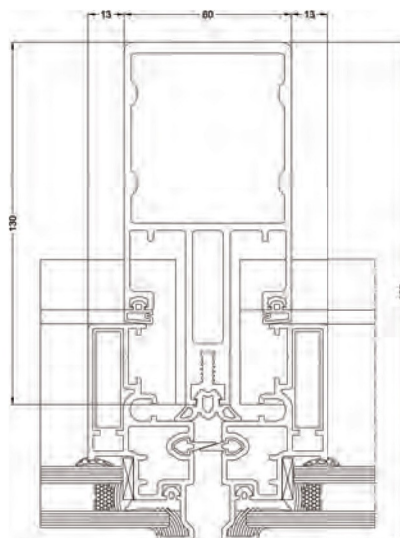
Facciate semistrutturali Semi structural curtain walls
